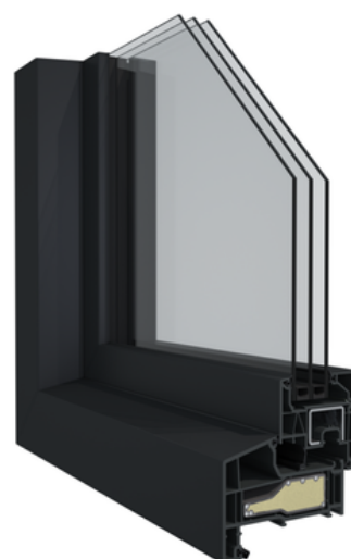
Grando (84 mm) możliwość zastosowania wzmocnienia termicznego Forthex.
